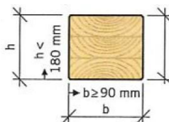
Limträpelare i hållfasthetsklass GL30h
