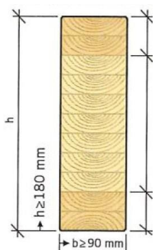
Limträbalk i hållfasthetsklass GL30c
